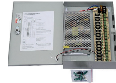
Fuente centralizada de 18CH 30AMP SAT PSV30A18CH
